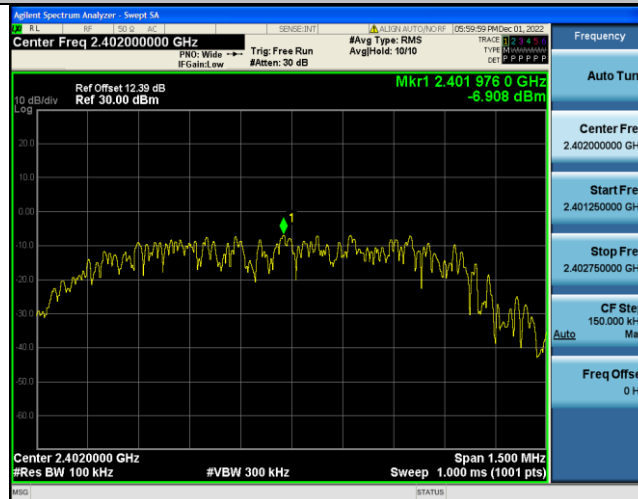
2DH5-Ant1-2402-30~1000--6.91
