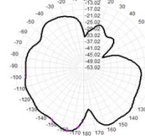
2500.0MHz Total(E2-YZ), Max=-16.22dB
