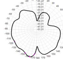
2490.0MHz Total(E2-YZ), Max=-13.02dB
