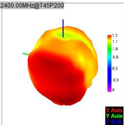
2450.00MHz@T45P200
