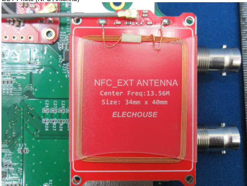
(16) EUT Photo (NFC Antenna)
