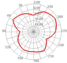
5150.000MHz E2
