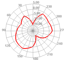
5150.000MHz E1
