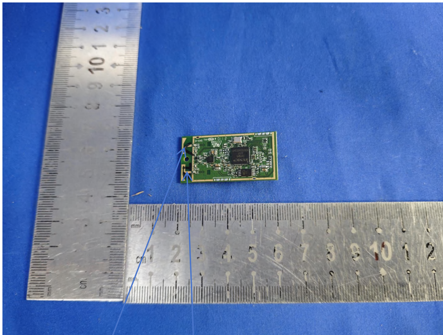
5.8G ANT 1 5.8G ANT 2
