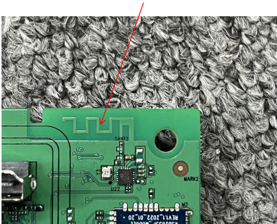
BLE Antenna
