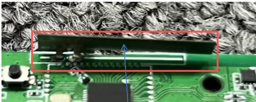
Antenna
