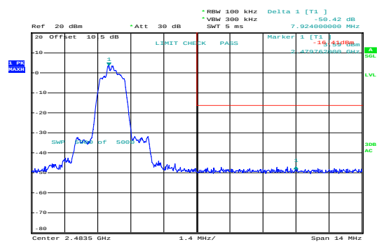
\pi/4 -DQPSK_High
