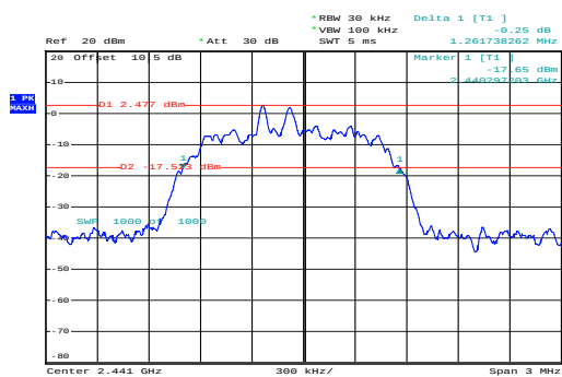
\pi/4 -DQPSK_Middle
