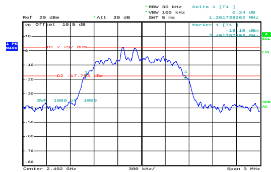
\pi/4 -DQPSK_Low
