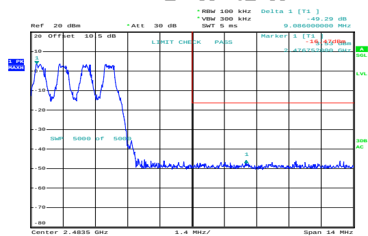
GFSK_Hopping_Upper
