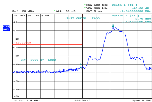
\pi/4 -DQPSK_Low
