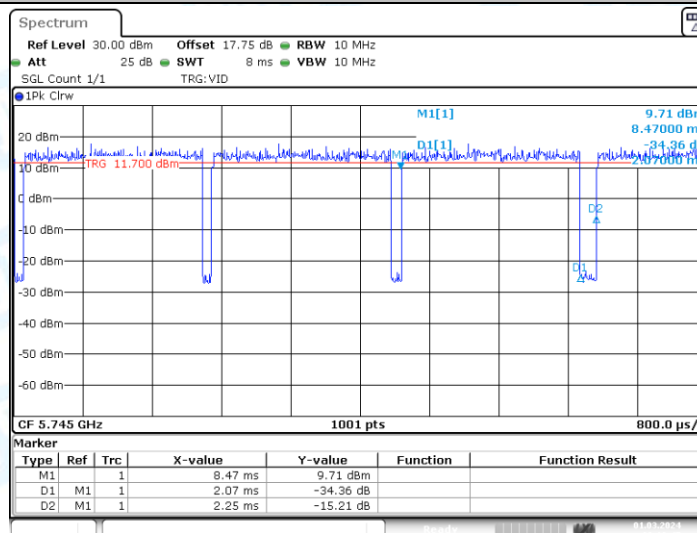
11A_Ant2_5745
