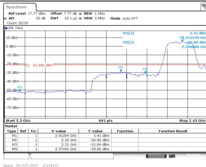
11N20MIMO_Ant2_Low_2412_AV
