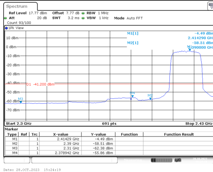
11N20MIMO_Ant1_Low_2412_Peak
