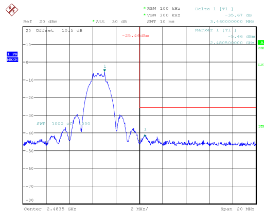
Right Side-2480MHz
