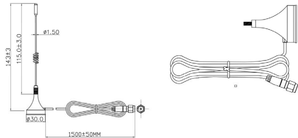
Lora antenna
