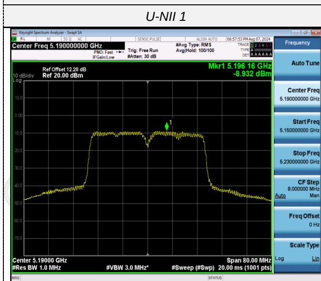
802.11ac(HT40)
