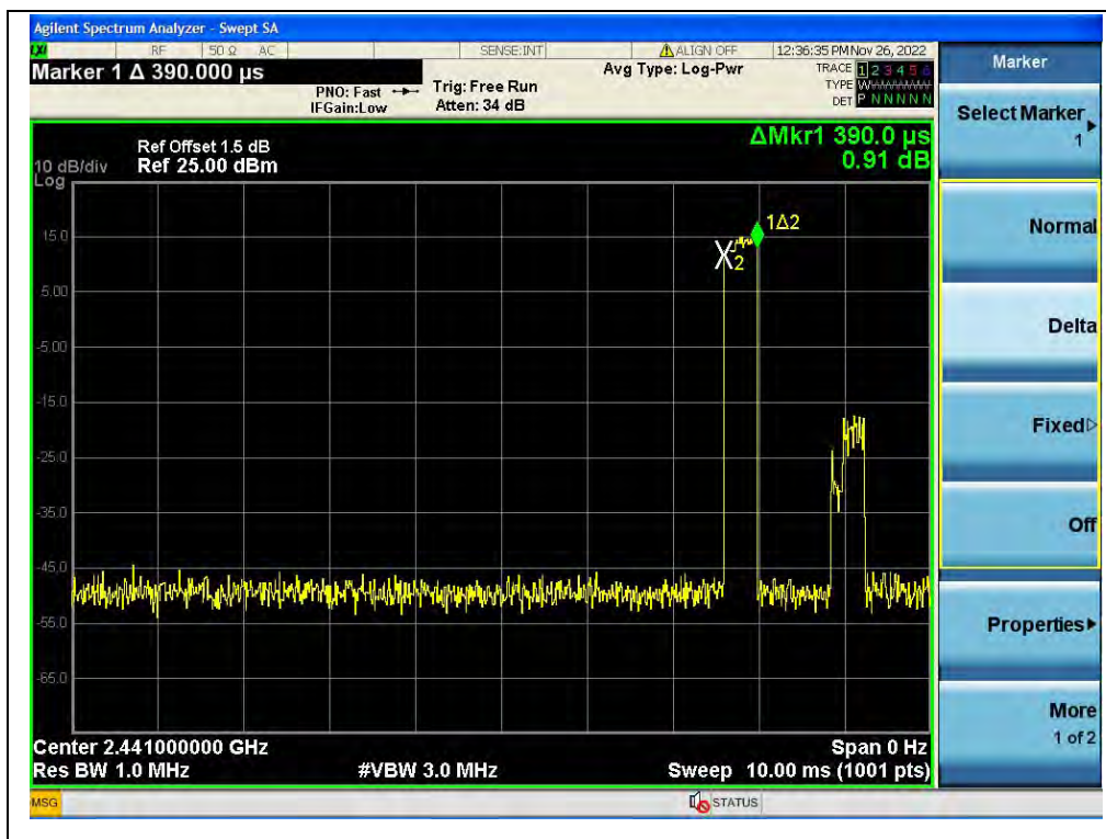
(DH1, 8-DPSK)
