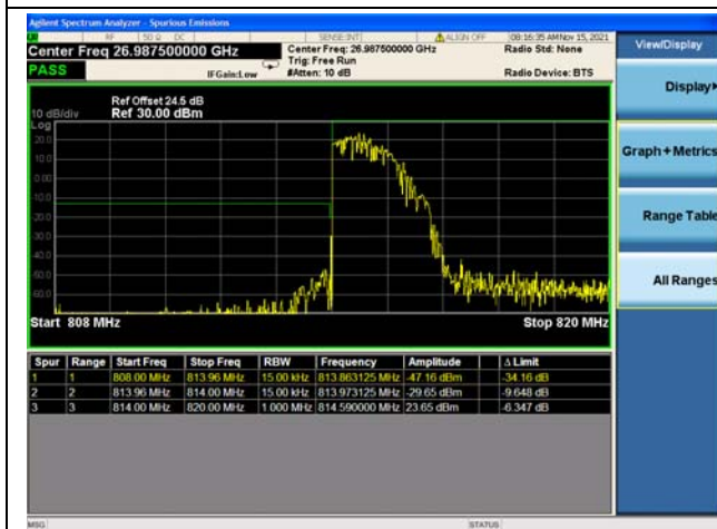
Band26 / 1.4MHz / Low CH / QPSK / 1 RB
