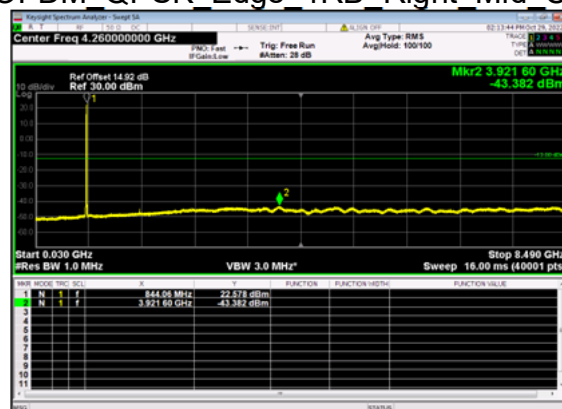
n5(15M)_DFT-s- OFDM QPSK Edge 1RB Right Mid CH
