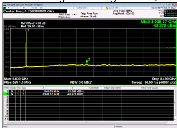
n5(20M)_DFT-s-OFDM_ BPSK Edge 1RB Right Mid CH
