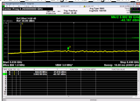
n5(20M)_DFT-s-OFDM BPSK Edge 1RB Right Low CH
