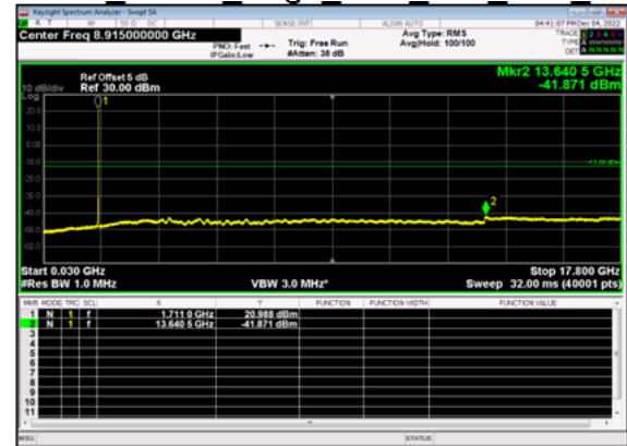
n66(10M)_DFT-s- OFDM QPSK Edge 1RB Left Low CH
