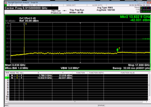
n66(10M)_DFT-s-OFDM QPSK Edge 1RB Right High CH
