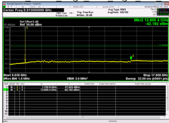
n66(15M)_DFT-s- OFDM BPSK Edge 1RB Right Mid CH
