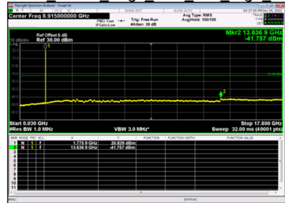
n66(5M)_DFT-s-OFDM QPSK Edge 1RB Left High CH
