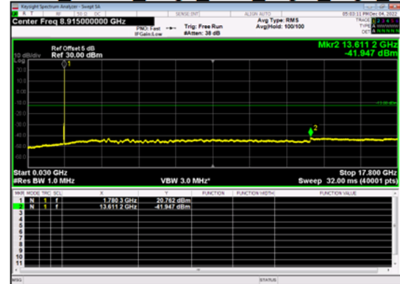
n66(15M)_DFT-s-OFDM QPSK Edge 1RB Right High CH
