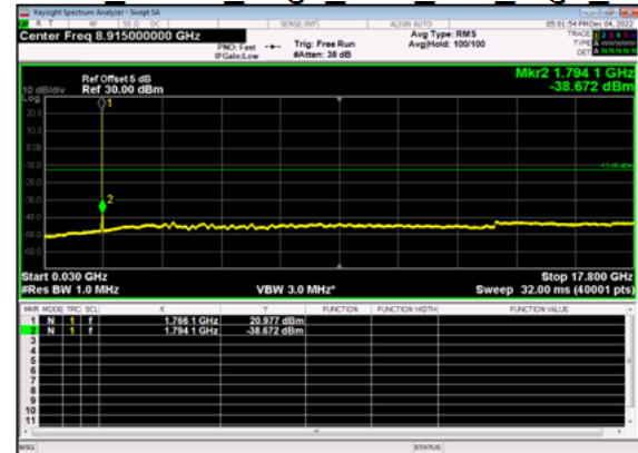
n66(15M)_DFT-s-OFDM QPSK Edge 1RB Left High CH
