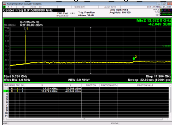
n66(10M)_DFT-s- OFDM BPSK Edge 1RB Right Low CH
