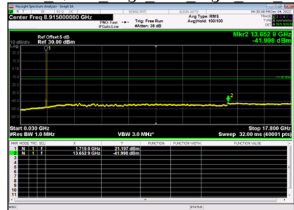
n66(5M)_DFT-s- OFDM QPSK Edge 1RB Right Low CH
