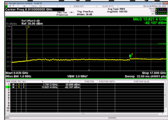
n66(20M)_DFT-s-OFDM QPSK Edge 1RB Left High CH
