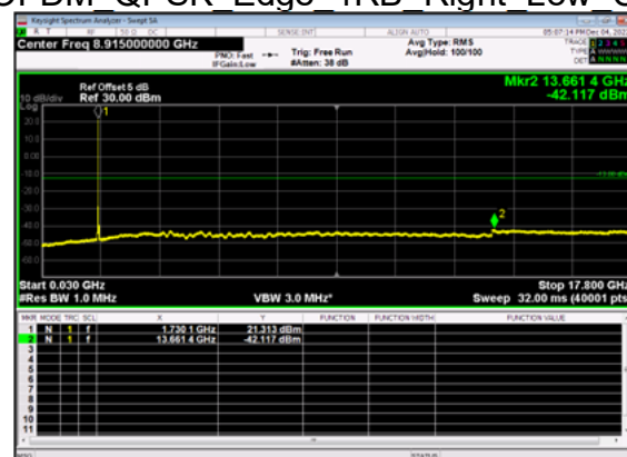
n66(20M)_DFT-s-OFDM QPSK Edge 1RB Right Low CH
