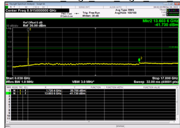
n66(10M)_DFT-s- OFDM QPSK Edge 1RB Right Low CH
