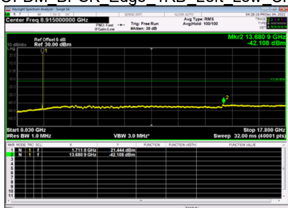
n66(5M)_DFT-s- OFDM BPSK Edge 1RB Left Low CH
