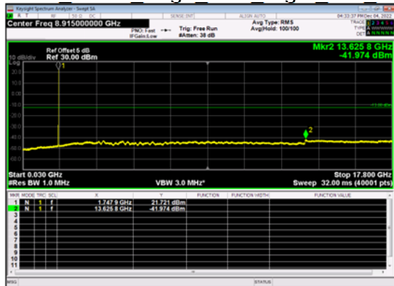
n66(5M)_DFT-s- OFDM BPSK Edge 1RB Right Mid CH
