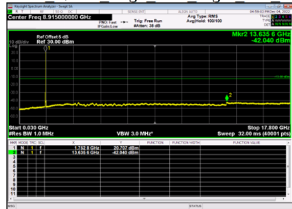
n66(15M)_DFT-s- OFDM QPSK Edge 1RB Right Mid CH
