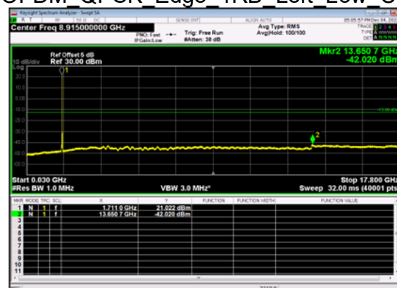
n66(20M)_DFT-s-OFDM QPSK Edge 1RB Left Low CH
