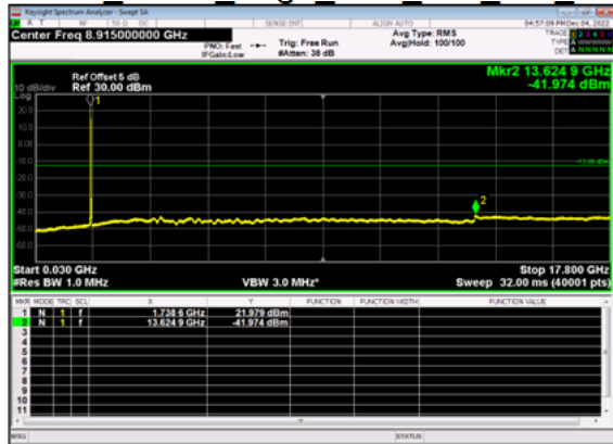
n66(15M)_DFT-s- OFDM BPSK Edge 1RB Left Mid CH
