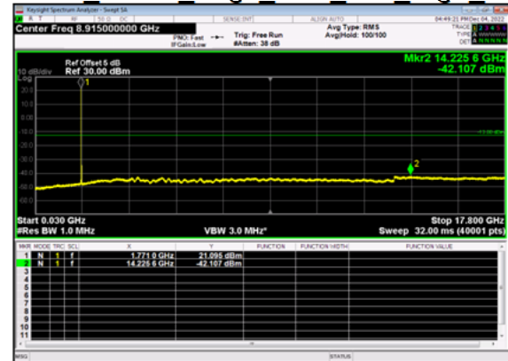
n66(10M)_DFT-s-OFDM QPSK Edge 1RB Left High CH
