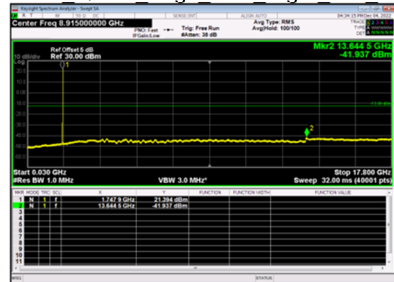
n66(5M)_DFT-s- OFDM QPSK Edge 1RB Right Mid CH
