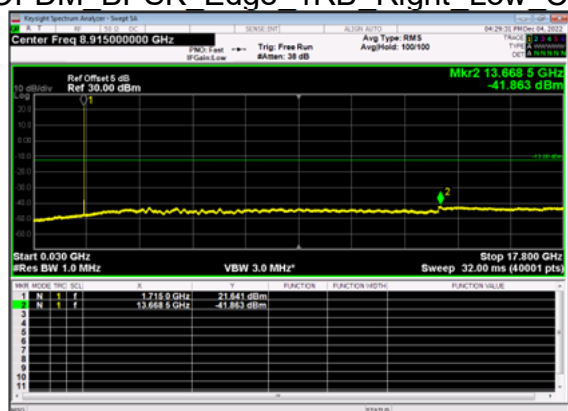
n66(5M)_DFT-s- OFDM BPSK Edge 1RB Right Low CH
