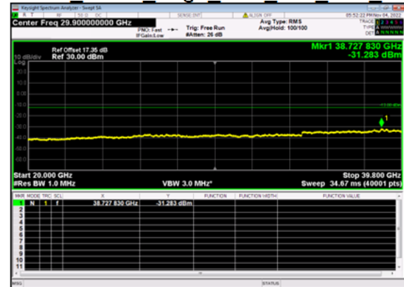
n77(60M)_DFT-s-OFDM BPSK Edge 1RB Left Low CH
