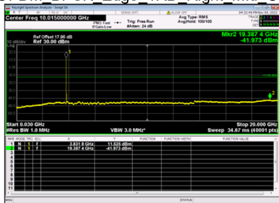
n77(20M)_DFT-s- OFDM BPSK Edge 1RB Right Mid CH
