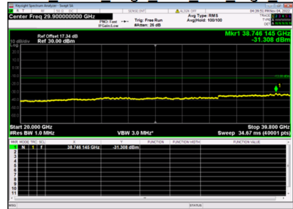
n77(20M)_DFT-s-OFDM BPSK Edge 1RB Left High CH
