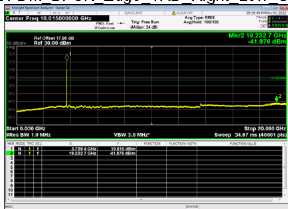
n77(40M)_DFT-s-OFDM BPSK Edge 1RB Right Low CH
