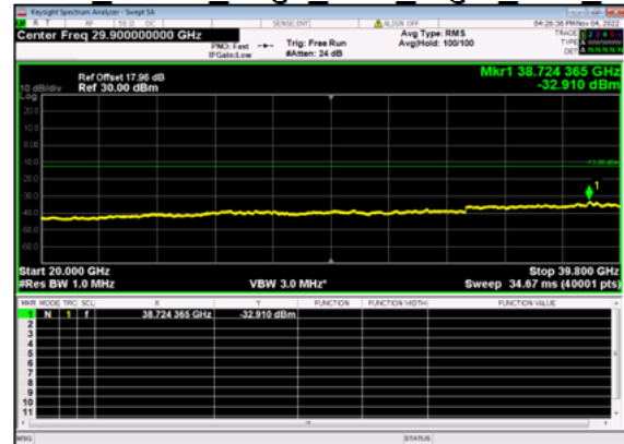
n77(20M)_DFT-s-OFDM QPSK Edge 1RB Right Low CH
