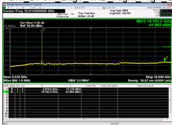
n77(20M)_DFT-s-OFDM BPSK Edge 1RB Right High CH
