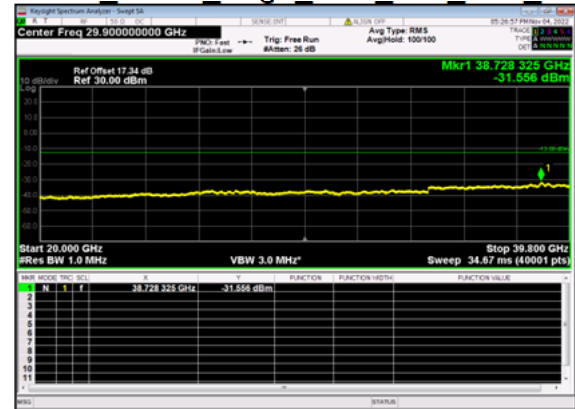
n77(40M)_DFT-s-OFDM BPSK Edge 1RB Left Low CH
