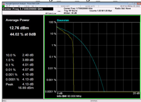
n77(60M)_DFT-s-OFDM_PI_2-BPSK Edge 1RB Right Low CH
