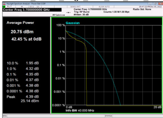
n77(40M)_DFT-s-OFDM QPSK Edge 1RB Left Low CH
