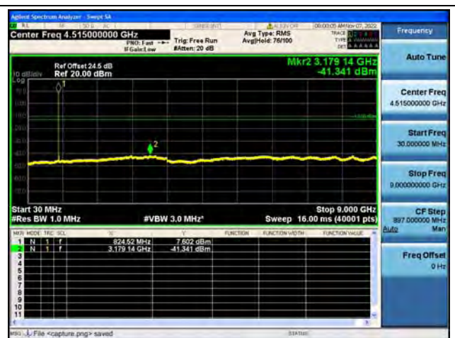
Band5 / 5MHz / Low CH / 16QAM
