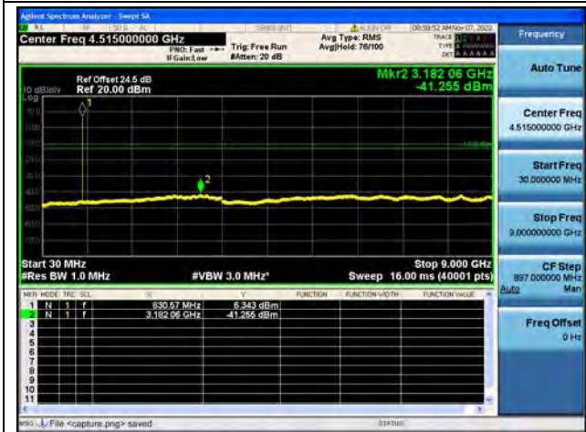
Band19 / 5MHz / Low CH / 64QAM
