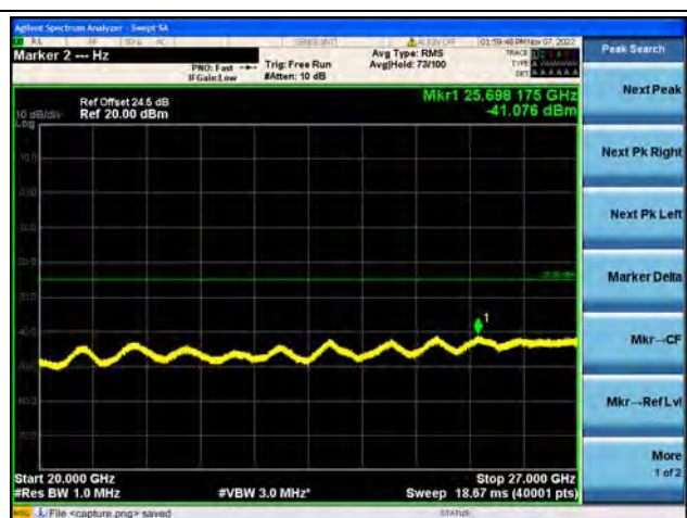
Band41-20G-27G / 10MHz / Mid CH / QPSK
