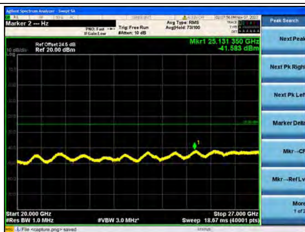
Band41-20G-27G / 20MHz / Mid CH / 16QAM
