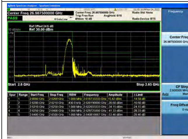
Band38 / 20MHz / High CH / QPSK / 1 RB
