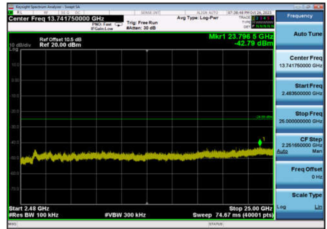
,Plot 4,2483.5MHz~25000MHz-802.11b ,2437MHz,Ant6
