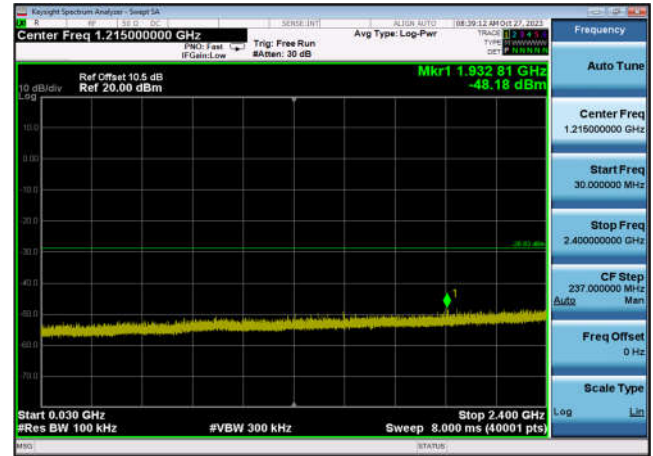
,Plot 3,30MHz~2400MHz-802.11n(HT20) ,2462MHz,Ant6
