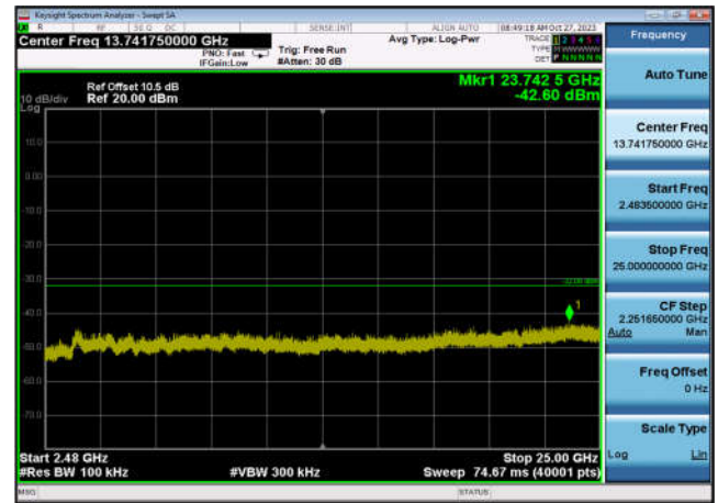
,Plot 4,2483.5MHz~25000MHz-802.11n(HT 40),2437MHz,Ant6
