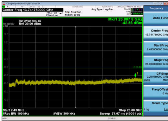
,Plot 4,2483.5MHz~25000MHz-802.11n(HT 40),2437MHz,Ant7
