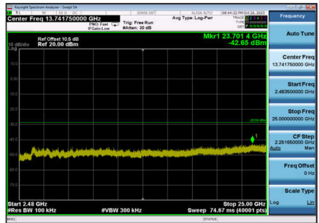
,Plot 4,2483.5MHz~25000MHz-802.11ax(HE20), 2462MHz,Ant6
