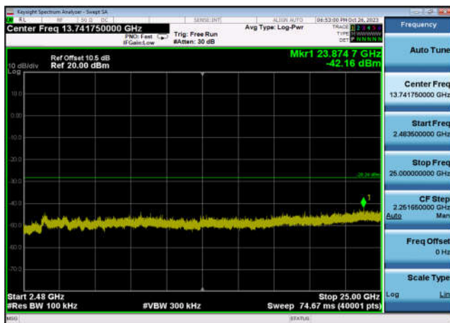
,Plot 4,2483.5MHz~25000MHz-802.11ax(HE20), 2462MHz,Ant7
