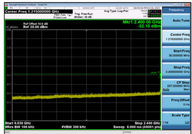
,Plot 3,30MHz~2400MHz-802.11ax(HE20) ,2437MHz,Ant6
