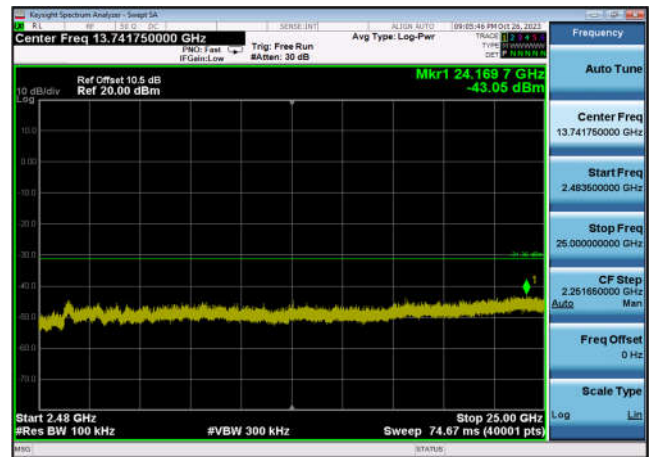
,Plot 4,2483.5MHz~25000MHz-802.11ax(HE40), 2452MHz,Ant6
