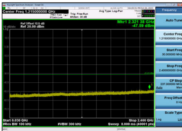
,Plot 3,30MHz~2400MHz-802.11n(HT40) ,2452MHz,Ant7
