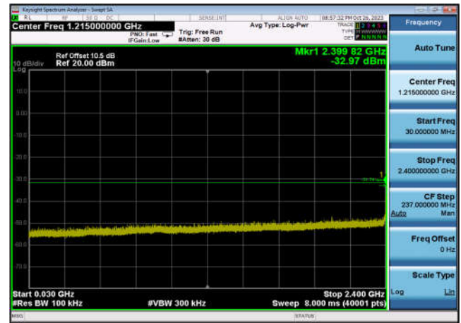
,Plot 3,30MHz~2400MHz-802.11ax(HE40) ,2437MHz,Ant6
