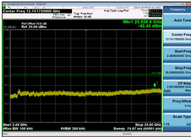
,Plot 4,2483.5MHz~25000MHz-802.11ax(HE20), 2437MHz,Ant7
