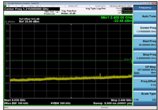
,Plot 3,30MHz~2400MHz-802.11n(HT20) ,2437MHz,Ant6
