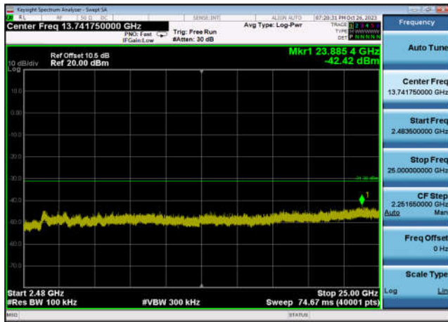
,Plot 4,2483.5MHz~25000MHz-802.11ax(HE40), 2437MHz,Ant7
