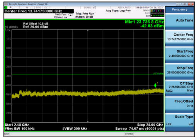
,Plot 4,2483.5MHz~25000MHz-802.11ax(HE20), 2437MHz,Ant6
