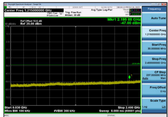
,Plot 3,30MHz~2400MHz-802.11ax(HE20) ,2462MHz,Ant6
