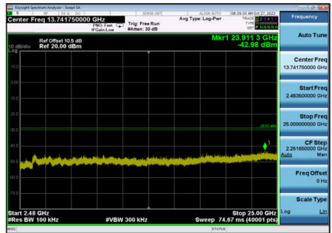
,Plot 4,2483.5MHz~25000MHz-802.11n(HT 20),2462MHz,Ant6
