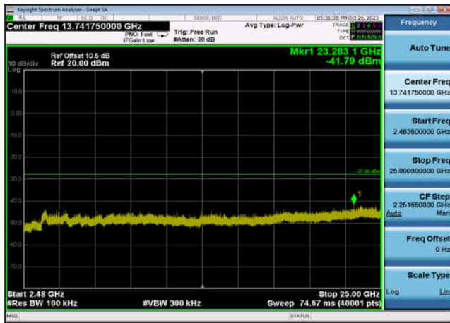
,Plot 4,2483.5MHz~25000MHz-802.11n(HT 20),2437MHz,Ant7
