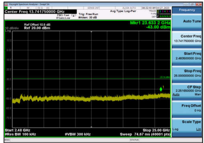
,Plot 4,2483.5MHz~25000MHz-802.11n(HT 20),2437MHz,Ant6
