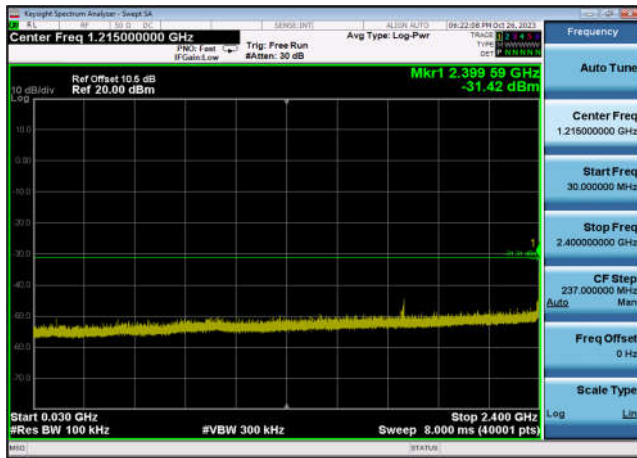
,Plot 3,30MHz~2400MHz-802.11n(HT40) ,2437MHz,Ant7
