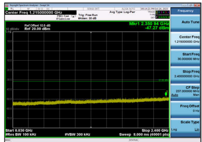
,Plot 3,30MHz~2400MHz-802.11ax(HE40) ,2452MHz,Ant6
