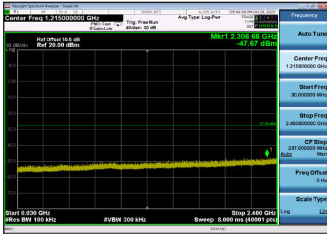
,Plot 3,30MHz~2400MHz-802.11n(HT20) ,2462MHz,Ant7
