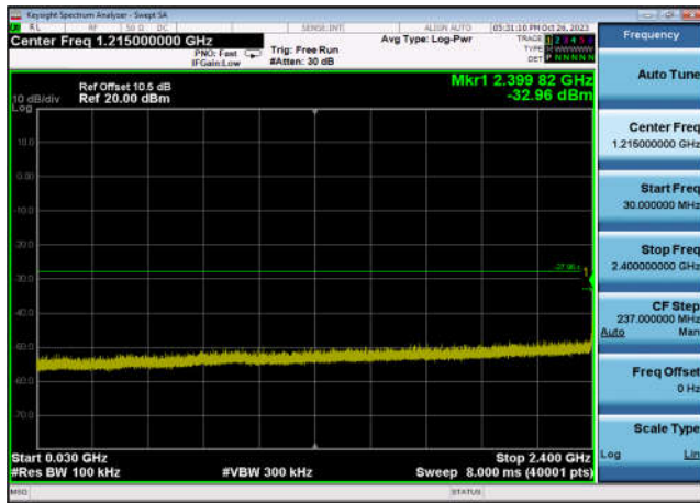
,Plot 3,30MHz~2400MHz-802.11n(HT20) ,2437MHz,Ant7
