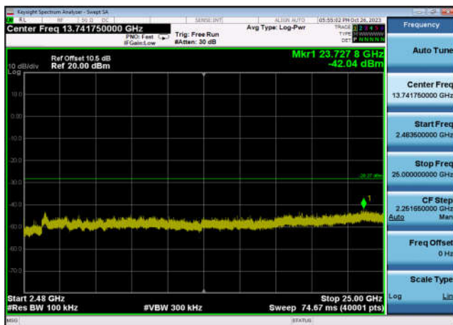
,Plot 4,2483.5MHz~25000MHz-802.11n(HT 20),2462MHz,Ant7
