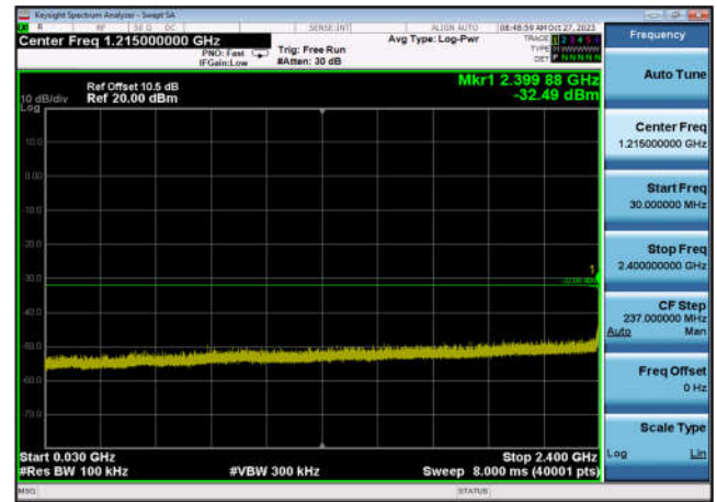
,Plot 3,30MHz~2400MHz-802.11n(HT40) ,2437MHz,Ant6
