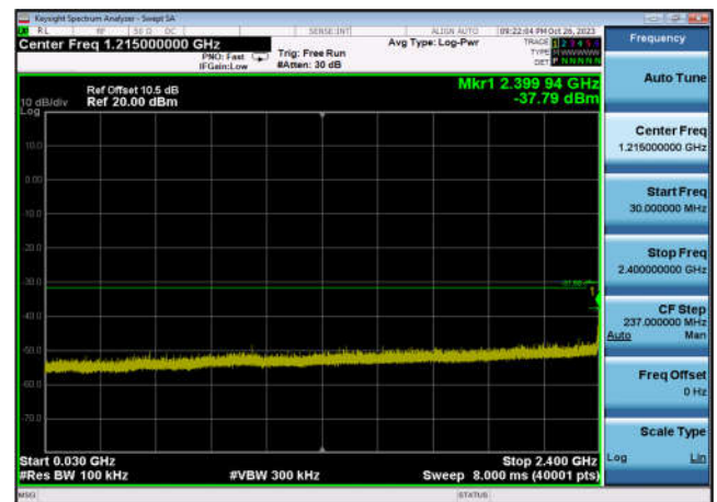
,Plot 3,30MHz~2400MHz-802.11n(HT40) ,2452MHz,Ant6
