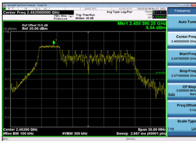
,Plot 1,Reference Level-802.11ax(HE20 _RU52_1),2462MHz,Ant6
