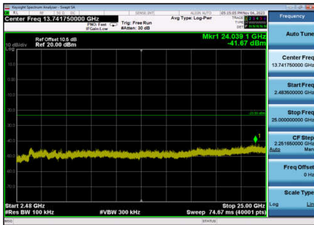
,Plot 4,2483.5MHz~25000MHz-802.11ax(H E20_RU52_4),2437MHz,Ant7
