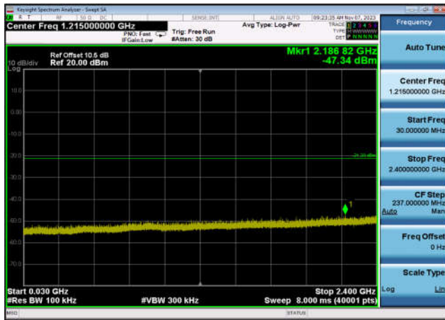
,Plot 3,30MHz~2400MHz-802.11ax(HE20 _RU26_9),2462MHz,Ant6
