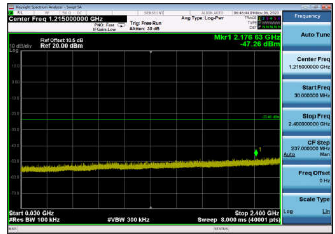
,Plot 3,30MHz~2400MHz-802.11ax(HE20 _RU52_4),2412MHz,Ant7
