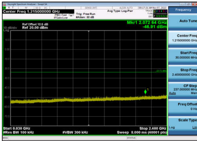
,Plot 3,30MHz~2400MHz-802.11ax(HE20 _RU52_4),2462MHz,Ant6
