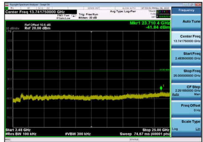
,Plot 4,2483.5MHz~25000MHz-802.11ax(H E20_RU26_9),2437MHz,Ant6
