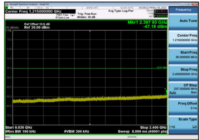
,Plot 3,30MHz~2400MHz-802.11ax(HE20 _RU26_9),2412MHz,Ant7
