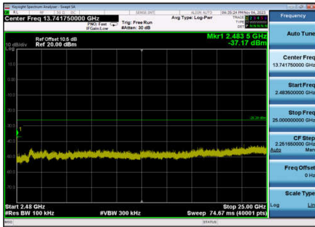
,Plot 4,2483.5MHz~25000MHz-802.11ax(H E20_RU26_1),2412MHz,Ant7
