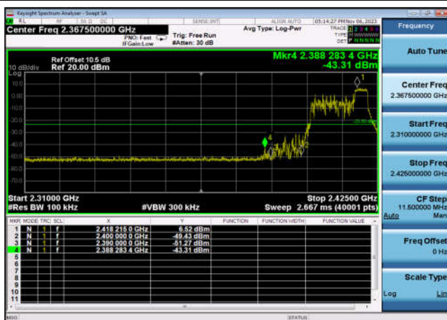
,Plot 2,Band Edge-802.11ax(HE20 _RU52_4),2412MHz,Ant7
