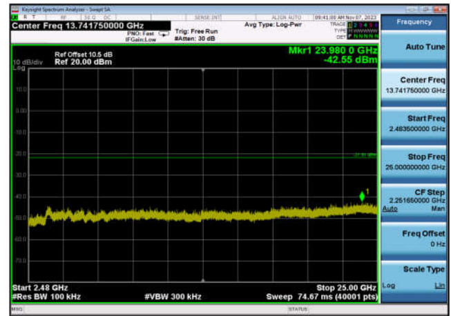
,Plot 4,2483.5MHz~25000MHz-802.11ax(H E20_RU26_9),2412MHz,Ant6
