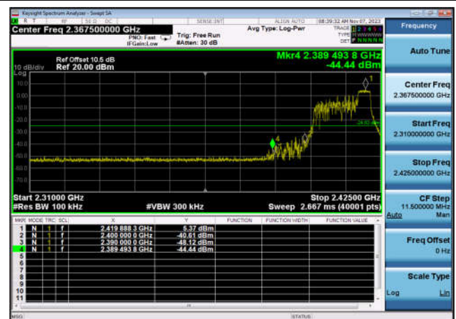
,Plot 2,Band Edge-802.11ax(HE20 _RU52_4),2412MHz,Ant6
