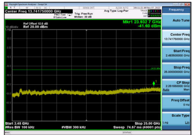
,Plot 4,2483.5MHz~25000MHz-802.11ax(H E20_RU52_1),2437MHz,Ant6
