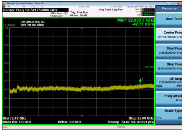
,Plot 4,2483.5MHz~25000MHz-802.11ax(H E20_RU106_2),2437MHz,Ant7
