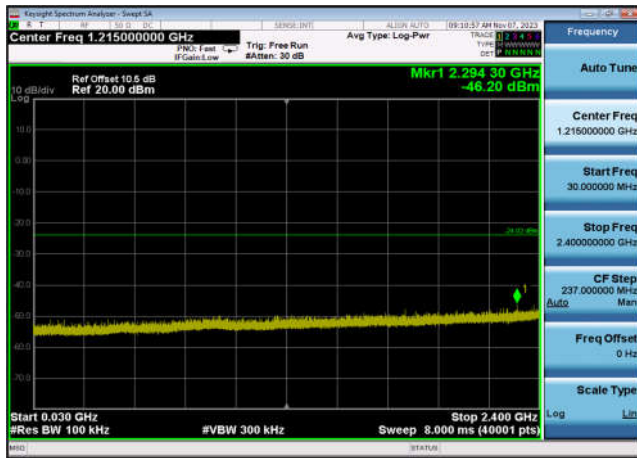
,Plot 3,30MHz~2400MHz-802.11ax(HE20 _RU52_1),2462MHz,Ant6
