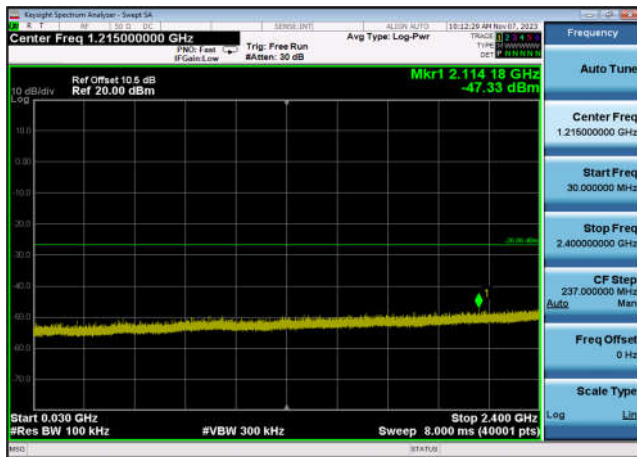
,Plot 3,30MHz~2400MHz-802.11ax(HE20 _RU26_1),2412MHz,Ant6
