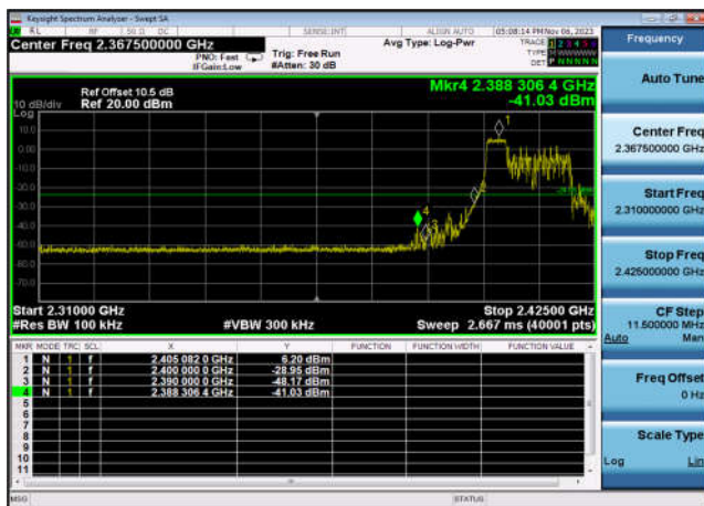
,Plot 2,Band Edge-802.11ax(HE20 _RU52_1),2412MHz,Ant7
