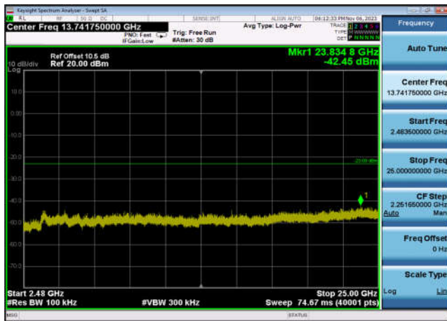
,Plot 4,2483.5MHz~25000MHz-802.11ax(H E20_RU52_1),2437MHz,Ant7
