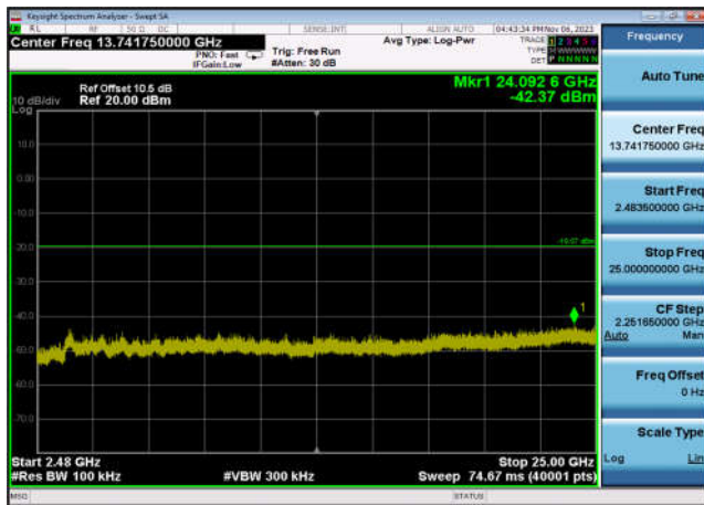
,Plot 4,2483.5MHz~25000MHz-802.11ax(H E20_RU26_9),2437MHz,Ant7
