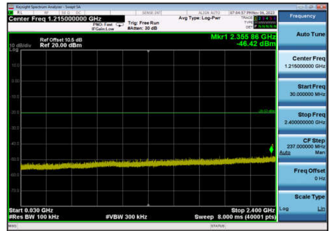
,Plot 3,30MHz~2400MHz-802.11ax(HE20 _RU52_1),2412MHz,Ant7
