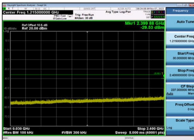
,Plot 3,30MHz~2400MHz-802.11ax(HE20 _RU52_1),2412MHz,Ant6
