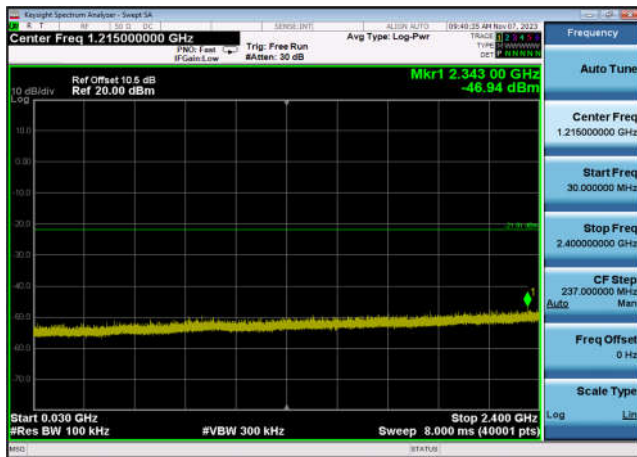
,Plot 3,30MHz~2400MHz-802.11ax(HE20 _RU26_9),2412MHz,Ant6
