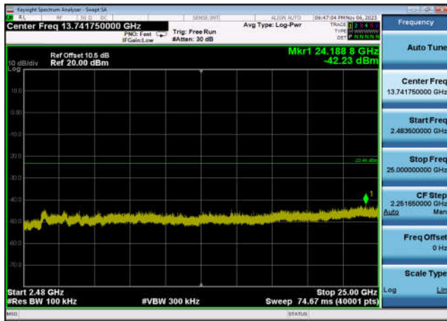
,Plot 4,2483.5MHz~25000MHz-802.11ax(H E20_RU52_4),2412MHz,Ant7
