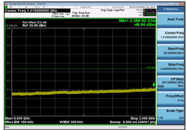
,Plot 3,30MHz~2400MHz-802.11ax(HE20 _RU26_1),2412MHz,Ant7
