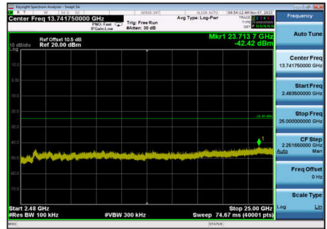
,Plot 4,2483.5MHz~25000MHz-802.11ax(H E20_RU52_4),2412MHz,Ant6
