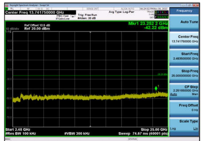
,Plot 4,2483.5MHz~25000MHz-802.11ax(H E20_RU106_1),2437MHz,Ant7
