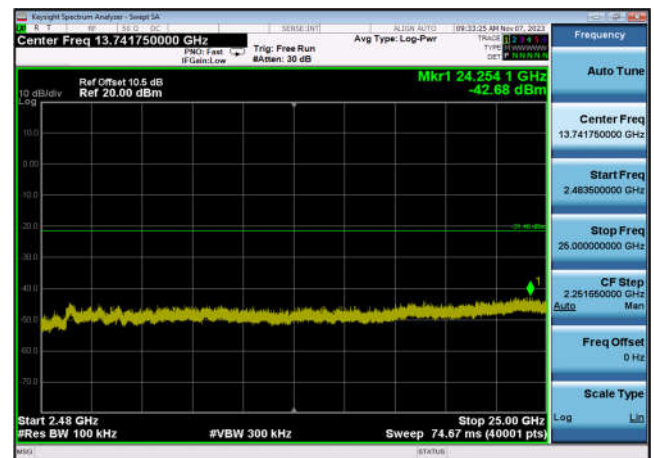
,Plot 4,2483.5MHz~25000MHz-802.11ax(H E20_RU26_1),2437MHz,Ant6
