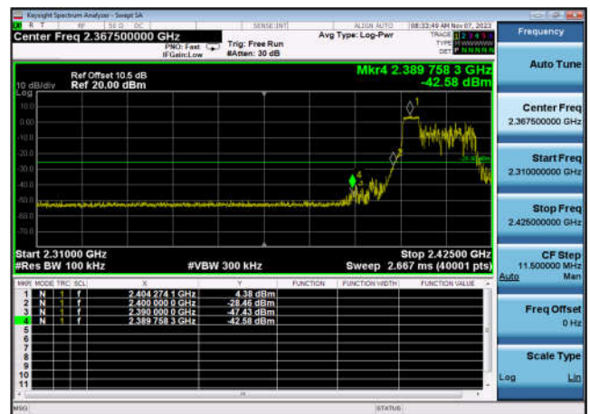
,Plot 2,Band Edge-802.11ax(HE20 _RU52_1),2412MHz,Ant6
