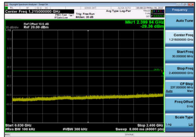
,Plot 3,30MHz~2400MHz-802.11ax(HE20 _RU52_1),2437MHz,Ant7
