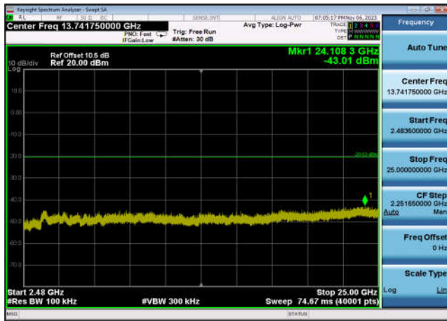
,Plot 4,2483.5MHz~25000MHz-802.11ax(H E20_RU52_1),2412MHz,Ant7
