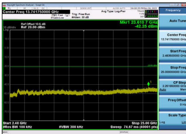
,Plot 4,2483.5MHz~25000MHz-802.11ax(H E20_RU26_1),2437MHz,Ant7
