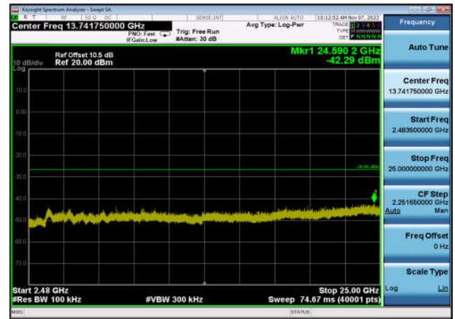
,Plot 4,2483.5MHz~25000MHz-802.11ax(H E20_RU26_1),2412MHz,Ant6
