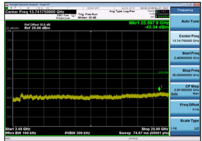
,Plot 4,2483.5MHz~25000MHz-802.11ax(H E20_RU52_4),2437MHz,Ant6
