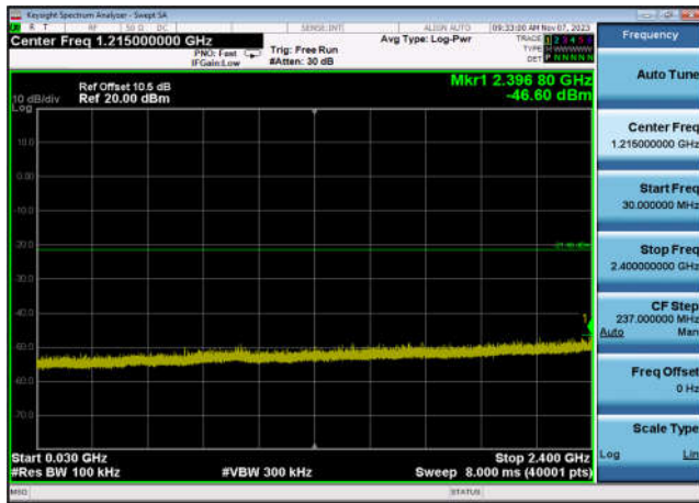
,Plot 3,30MHz~2400MHz-802.11ax(HE20 _RU26_1),2462MHz,Ant6
