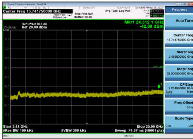
,Plot 4,2483.5MHz~25000MHz-802.11ax(H E20_RU26_9),2412MHz,Ant7
