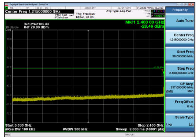
,Plot 3,30MHz~2400MHz-802.11ax(HE20 _RU26_1),2437MHz,Ant7
