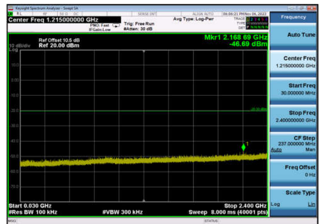
,Plot 3,30MHz~2400MHz-802.11ax(HE20 _RU26_9),2437MHz,Ant7
