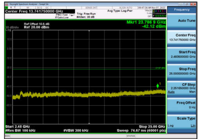
,Plot 4,2483.5MHz~25000MHz-802.11ax(H E20_RU52_1),2412MHz,Ant6
