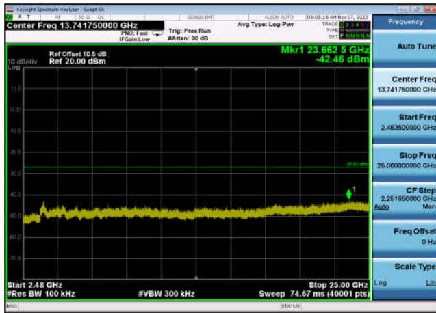
,Plot 4,2483.5MHz~25000MHz-802.11ax(H E20_RU106_2),2412MHz,Ant7
