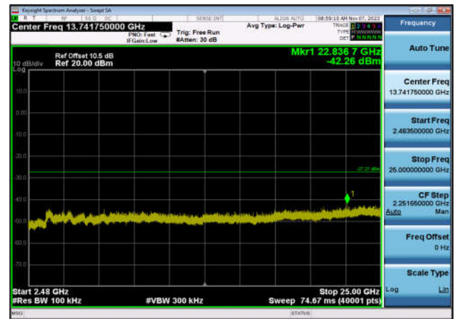
,Plot 4,2483.5MHz~25000MHz-802.11ax(H E20_RU106_2),2437MHz,Ant6
