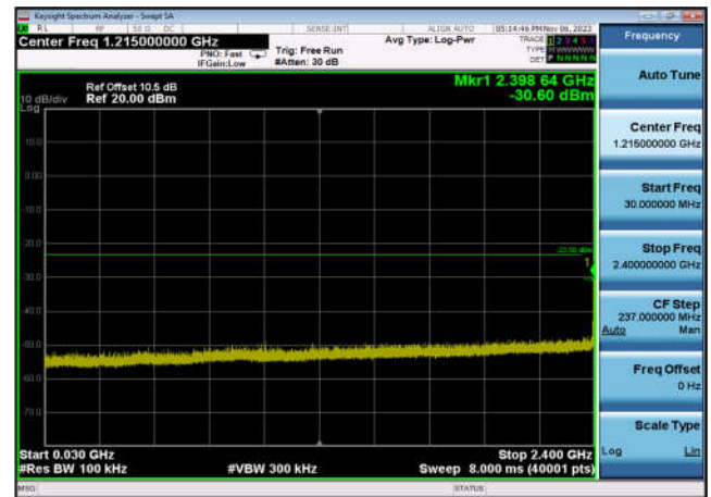
,Plot 3,30MHz~2400MHz-802.11ax(HE20 _RU52_4),2437MHz,Ant7
