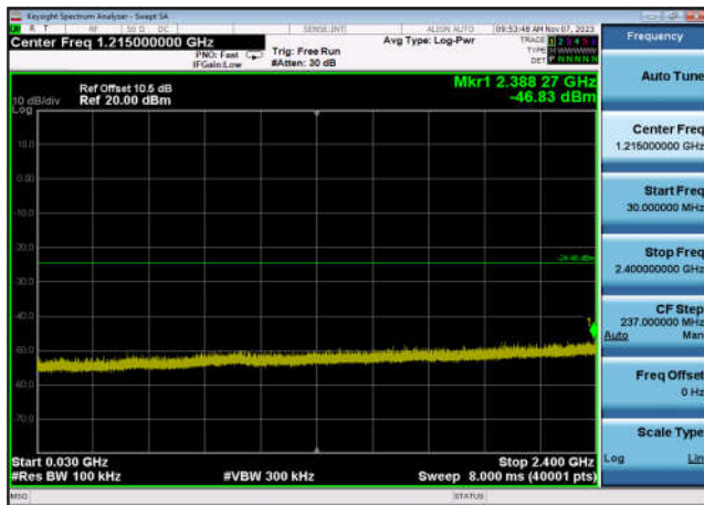
,Plot 3,30MHz~2400MHz-802.11ax(HE20 _RU52_4),2412MHz,Ant6
