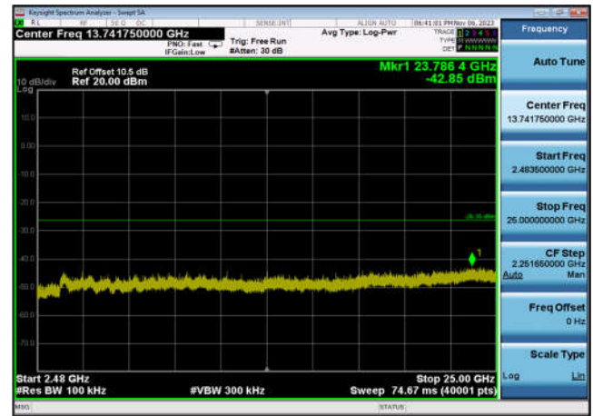
,Plot 4,2483.5MHz~25000MHz-802.11ax(H E20_RU106_2),2412MHz,Ant6
