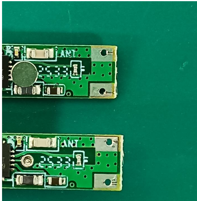
Antenna
