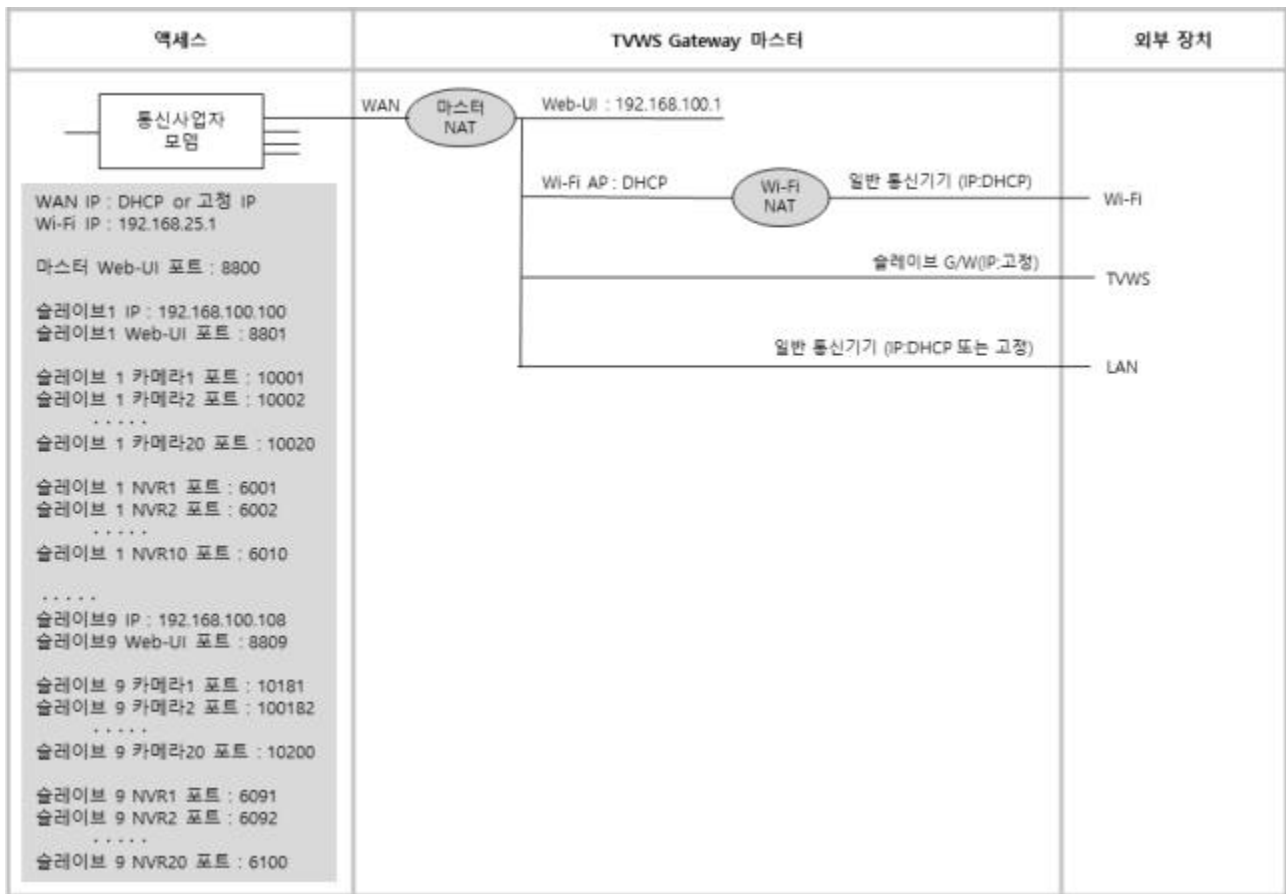
그림 4. TVWS Gateway 마스터 네트워크 구성도
