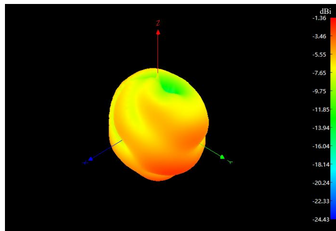
2450MHz 3D
