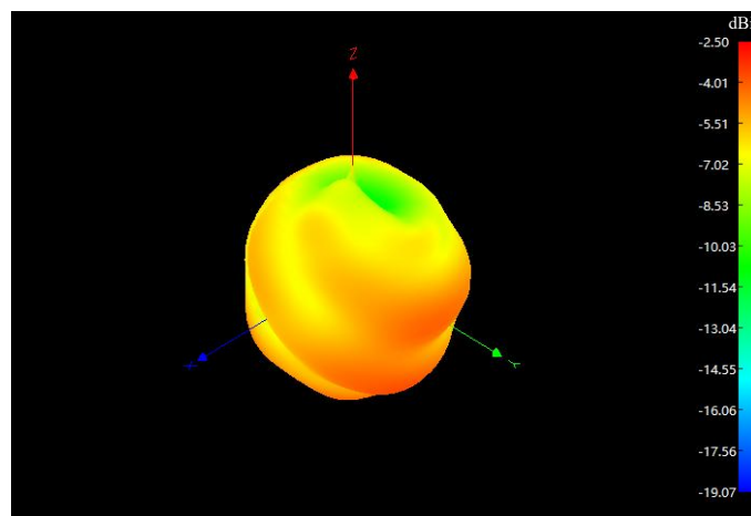
2500MHz 3D
