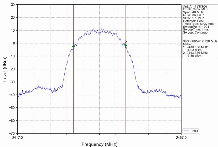
802.11b_MCH_2437MHz_Ant1 (SISO)_NTNV
