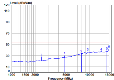
BLE_2M_TX_CH_00_Vertical-Avg
