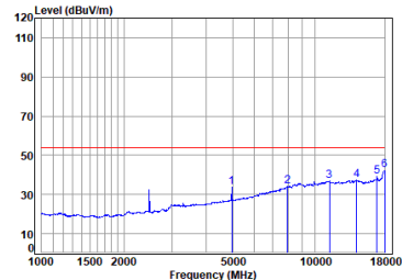
BLE_2M_TX_CH_39_Vertical-Avg
