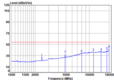
BLE_2M_TX_CH_19_Vertical-Avg
