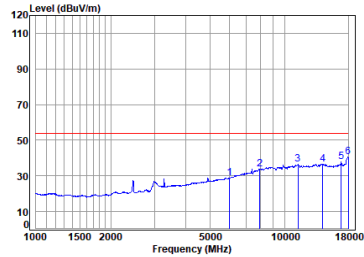
11n_20M_TX_CH_11_Horizontal-Avg
