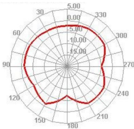
2450.000MHz E2
