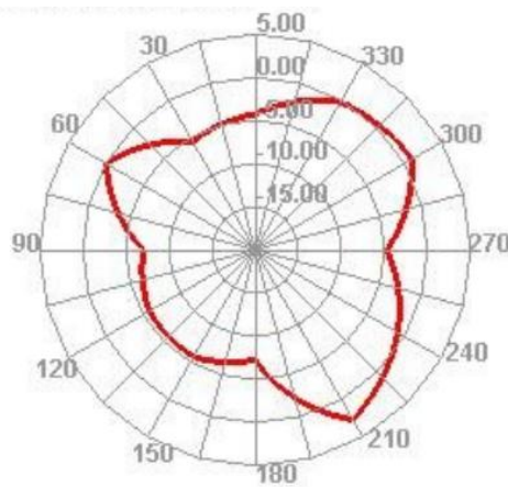
2400.000MHz E2
