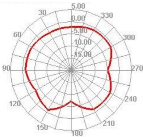
2500.000MHz E2
