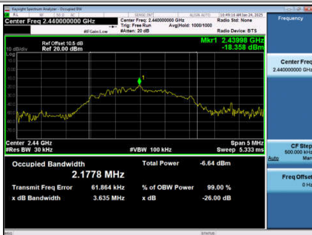
BLE_2M-Ant1-2440
