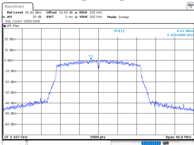
802.11n20_2437MHz_Chain 1
