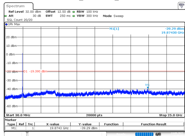
802.11n20_2437MHz_Chain 1
