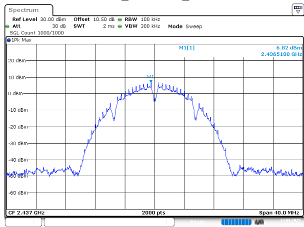
802.11b_2437MHz_Chain 1
