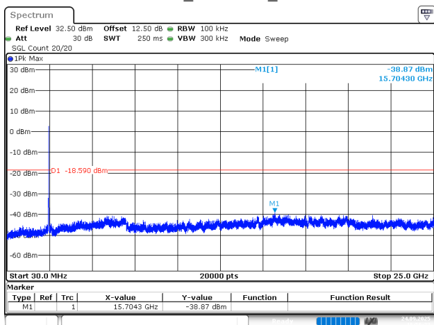
802.11n20_2462MHz_Chain 1
