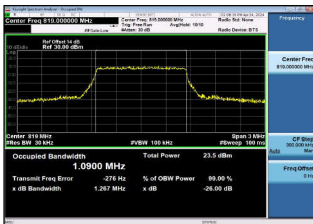
FDD26_Part 90_MidRange_10_819_Q16
