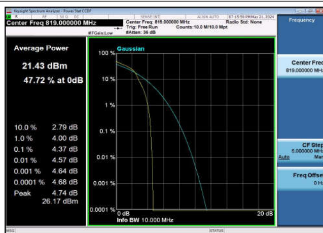
FDD26_Part 90_MidRange_10MHz_819_OneRB_high_Q16
