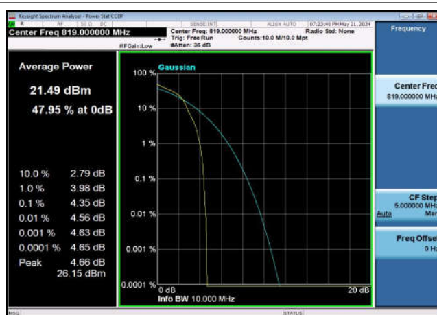
FDD26_Part 90_LowRange_10MHz_819_OneRB_high_Q16
