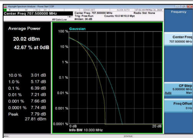
FDD12_MidRange_10MHz_707.5_fullIRB _Q16
