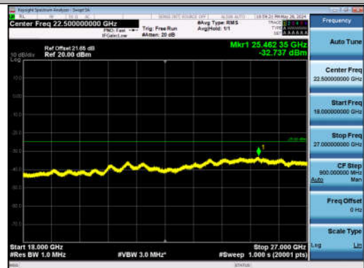
7-7-20MHz-20MHz-QPSK-QPSK-20850-21048-1RB#0-0RB #0-18000~27000MHz-PASS
