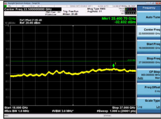
7-7-20MHz-20MHz-QPSK-QPSK-21001-21199-1RB#0-0RB #0-18000~27000MHz-PASS
