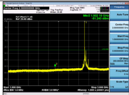
7-7-20MHz-20MHz-QPSK-QPSK-21001-21199-1RB#0-0RB #0-1000~3000MHz-PASS
