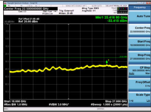
41-41-20MHz-20MHz-QPSK-QPSK-40641-40839-1RB#0-0 RB#0-18000~27000MHz-PASS
