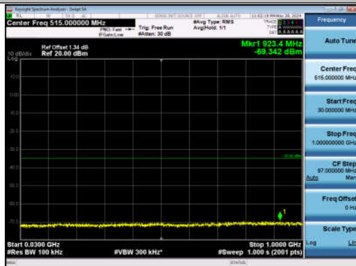
7-7-20MHz-20MHz-QPSK-QPSK-21001-21199-1RB#0-0R B#0-30~1000MHz-PASS
