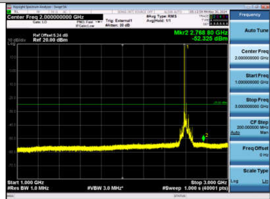
41-41-20MHz-20MHz-QPSK-QPSK-40641-40839-1RB#0-0 RB#0-1000~3000MHz-PASS
