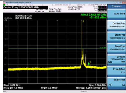
7-7-20MHz-20MHz-QPSK-QPSK-20850-21048-1RB#0-0RB #0-1000~3000MHz-PASS
