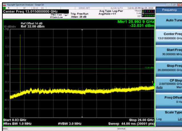
FDD25_HighRange_20MHz_30MHz~26GHz
