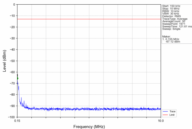
Band2_1.4MHz_QPSK_HCH_1909.3MHz_RB_1_0_NTNV
