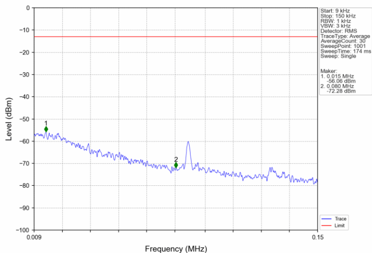
Band2_1.4MHz_QPSK_HCH_1909.3MHz_RB_1_0_NTNV
