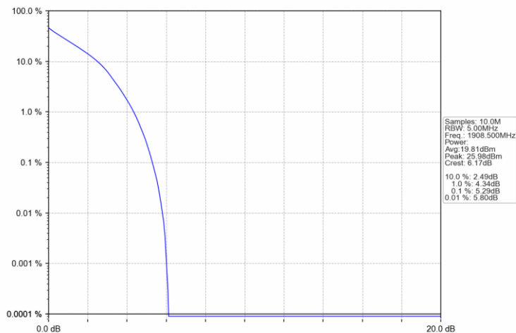
Band2_3MHz_QPSK_HCH_1908.5MHz_RB_15_0_NTNV
