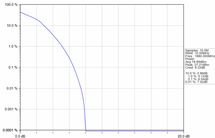
Band2_10MHz_16QAM_MCH_1880MHz_RB_50_0_NTNV
