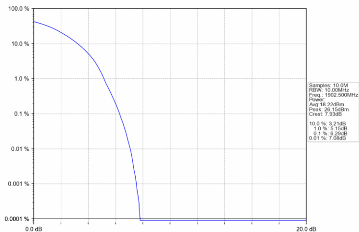
Band2 15MHz 16QAM HCH 1902.5MHz RB 75 0 NTV
