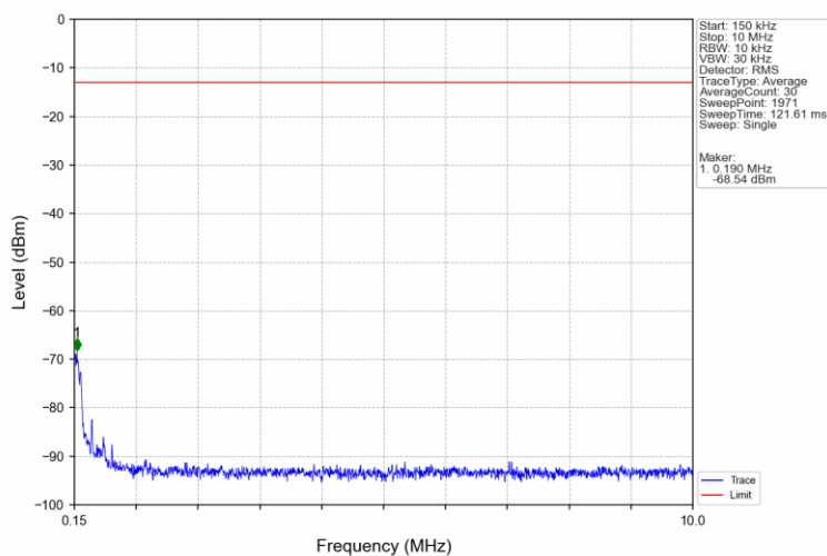
Band2 5MHz 16QAM LCH 1852.5MHz RB 1 0 NTV
