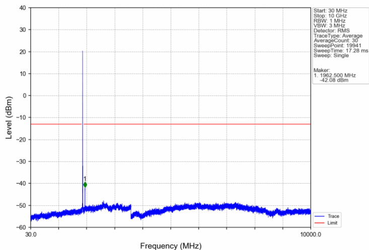
Band2 5MHz QPSK MCH 1880MHz RB 1 0 NTNV
