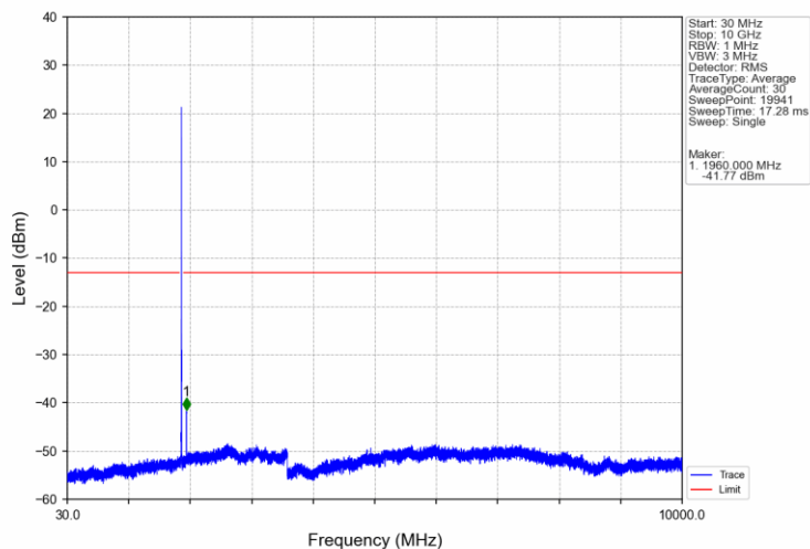
Band2_3MHz_QPSK_MCH_1880MHz_RB_1_0_NTNV
