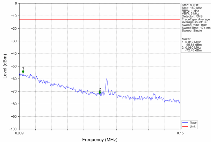
Band2_3MHz_16QAM_MCH_1880MHz_RB_1_0_NTNV
