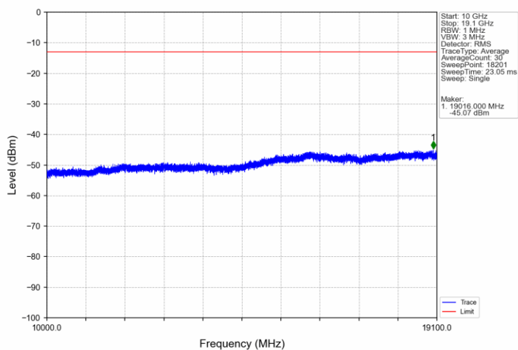
Band2 5MHz QPSK MCH 1880MHz RB 1 0 NTNV
