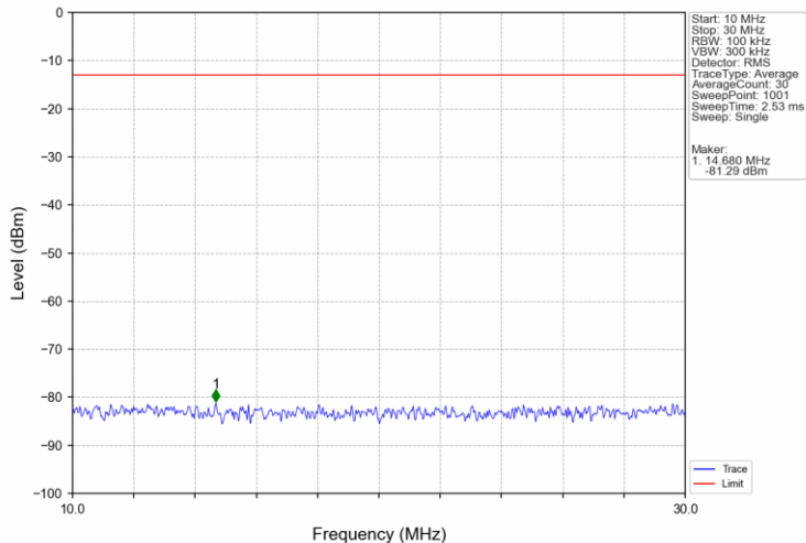
Band2_10MHz_16QAM_LCH_1855MHz_RB_1_0_NTNV
