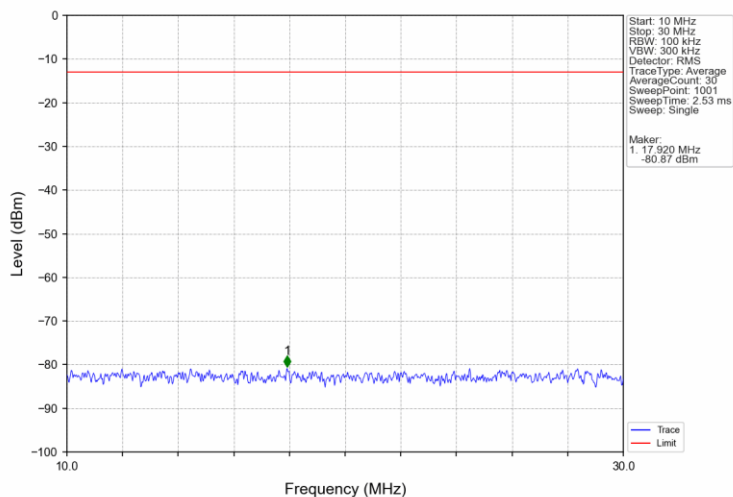
Band2_20MHz_QPSK_HCH_1900MHz_RB_1_0_NTNV
