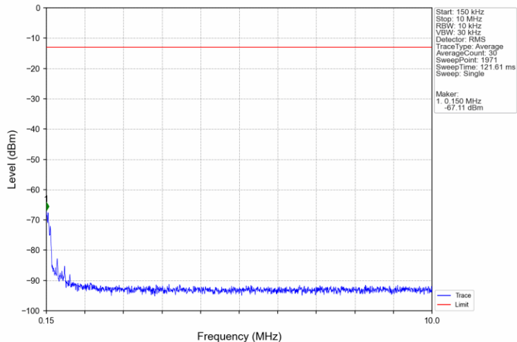
Band2_20MHz_QPSK_LCH_1860MHz_RB_1_0_NTNV
