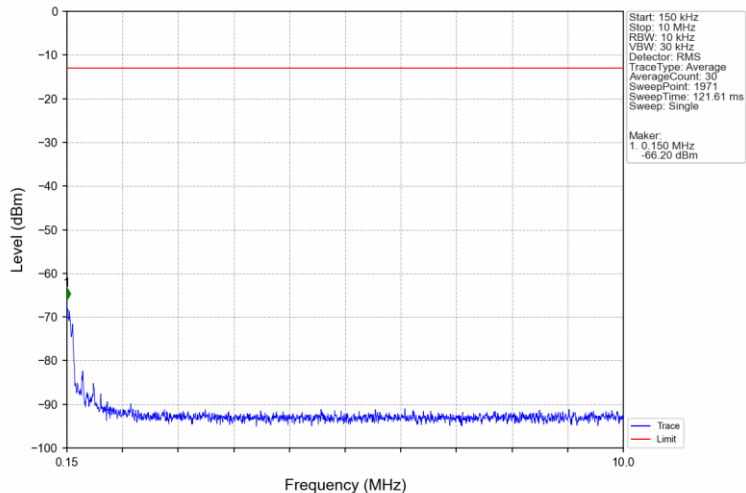
Band2_20MHz_QPSK_MCH_1880MHz_RB_1_0_NTNV
