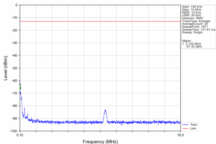
Band4 20MHz QPSK LCH 1720MHz RB 1 0 NTNV
