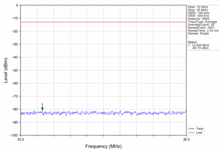
Band4 20MHz QPSK LCH 1720MHz RB 1 0 NTNV
