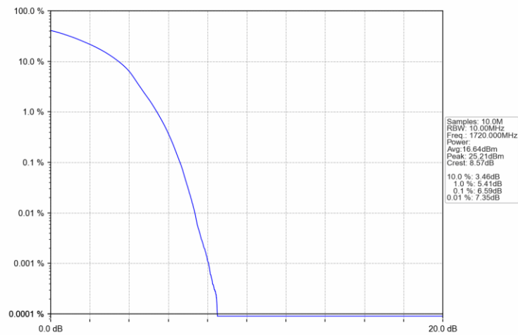
Band66 20MHz 16QAM LCH 1720MHz RB 100 0 NTNV
