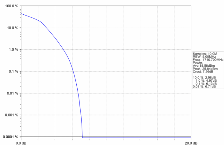
Band66 1.4MHz 16QAM LCH 1710.7MHz RB 6 0 NTNV
