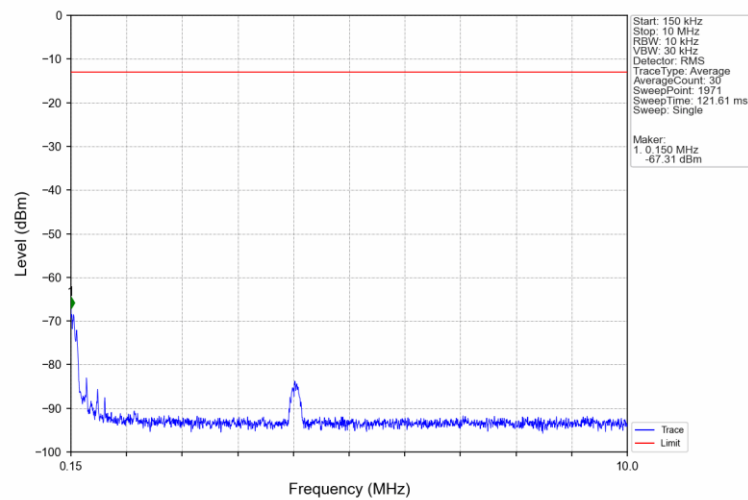
Band66 1.4MHz 16QAM LCH 1710.7MHz RB 1 0 NTNV
