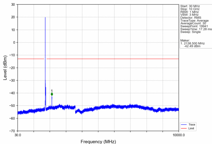
Band66_20MHz_QPSK_MCH_1745MHz_RB_1_0_NTNV
