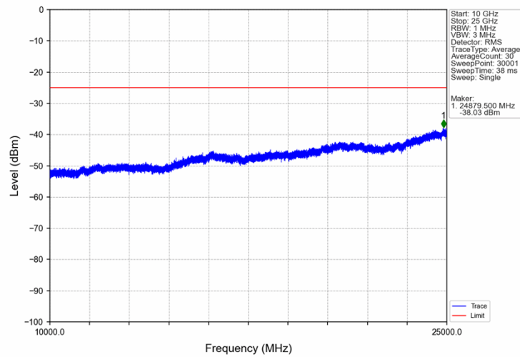
Band7 5MHz QPSK LCH 2502.5MHz RB 1 0 NTNV
