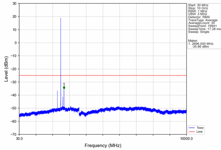
Band7 5MHz QPSK LCH 2502.5MHz RB 1 0 NTNV
