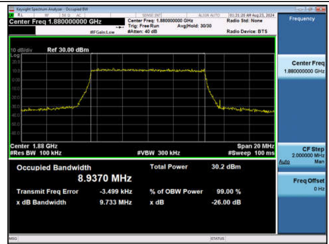
Band2-10MHz-16QAM-18900-50RB#0-PASS
