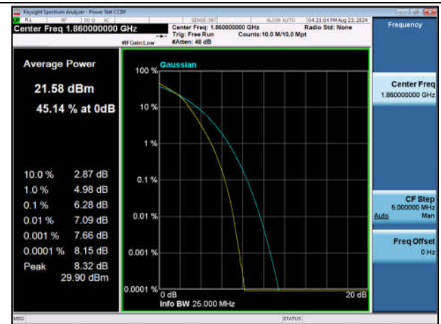
Band2-20MHz-16QAM-18700-100RB#0-PASS
