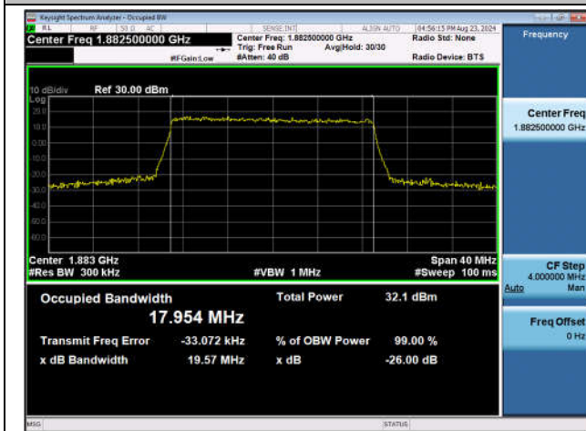
Band25-20MHz-QPSK-26365-100RB#0-PASS
