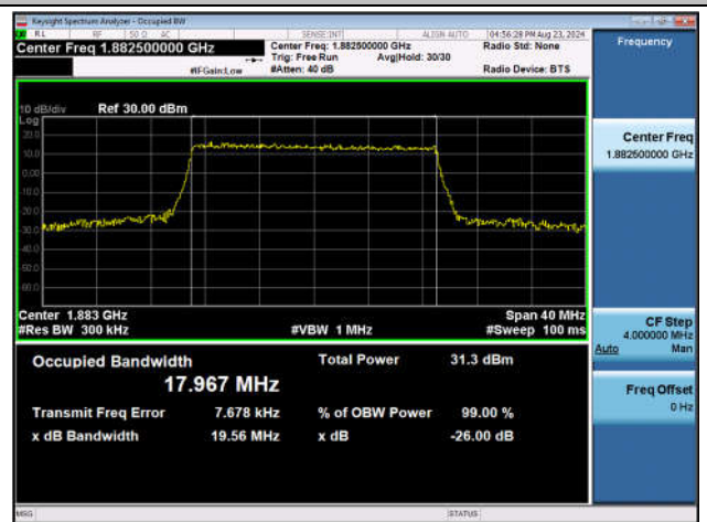
Band25-20MHz-16QAM-26365-100RB#0-PASS
