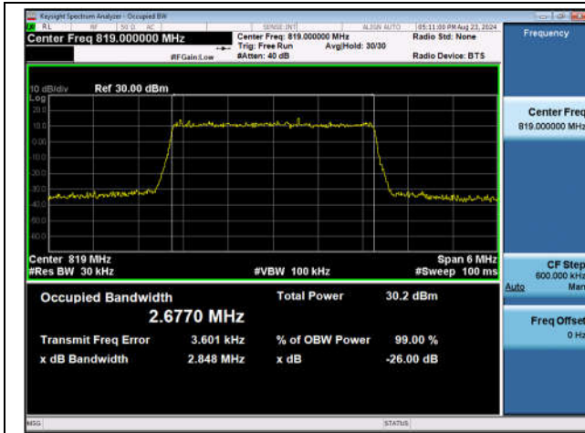
Band26(Part 90)-3MHz-QPSK-26740-15RB#0-PASS
