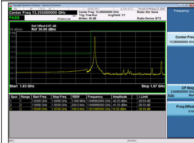
Band2_20MHz_QPSK_18700_1RB#0
