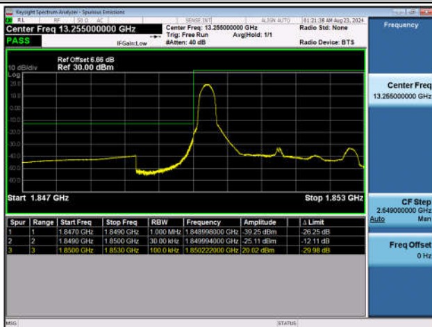
Band2_3MHz_QPSK_18615_1RB#0
