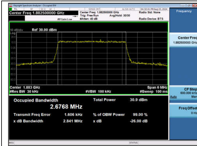
Band25-3MHz-QPSK-26365-15RB#0-PASS
