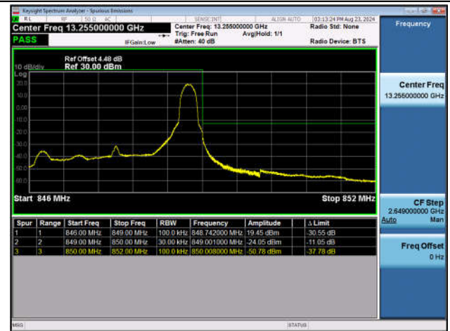
Band5_3MHz_QPSK_20635_1RB#14
