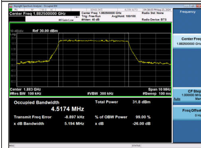
Band25-5MHz-QPSK-26365-25RB#0-PASS
