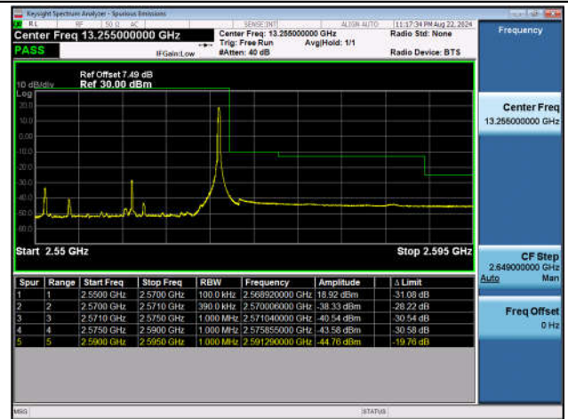
Band7_20MHz_QPSK_21350_1RB#99
