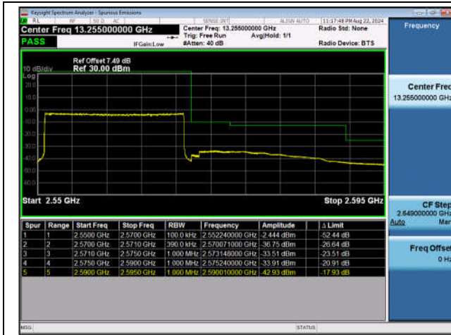
Band7_20MHz_QPSK_21350_100RB#0
