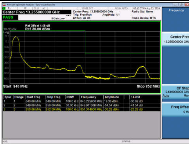
Band5_3MHz_QPSK_20635_1RB#0
