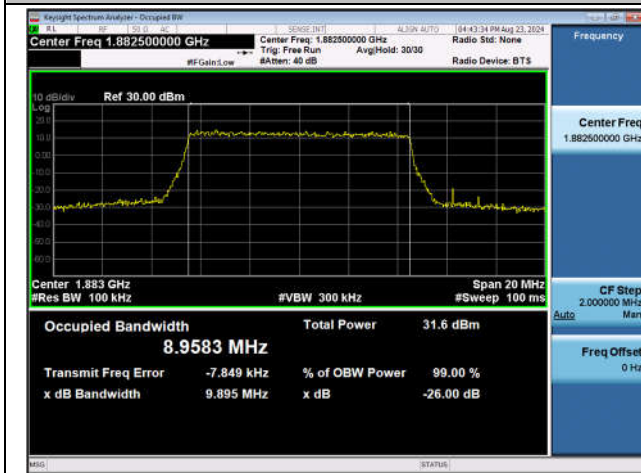
Band25-10MHz-QPSK-26365-50RB#0-PASS
