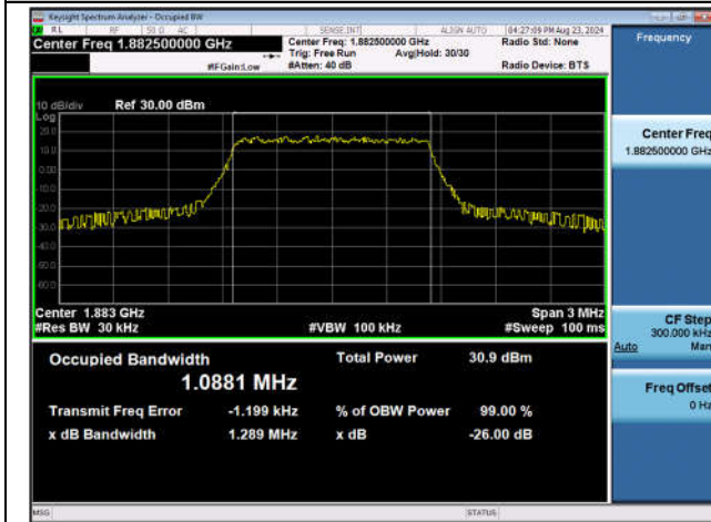
Band25-1.4MHz-QPSK-26365-6RB#0-PASS
