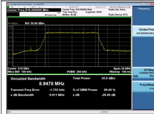
Band26(Part 90)-10MHz-QPSK-26740-50RB#0-PASS
