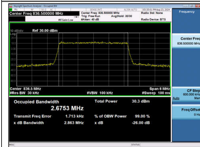
Band26(Part 22)-3MHz-QPSK-26915-15RB#0-PASS
