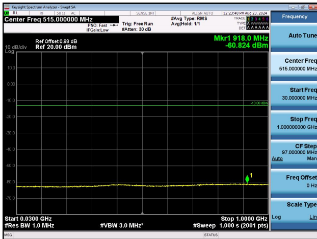
Band4-1312-30~1000MHz-PASS
