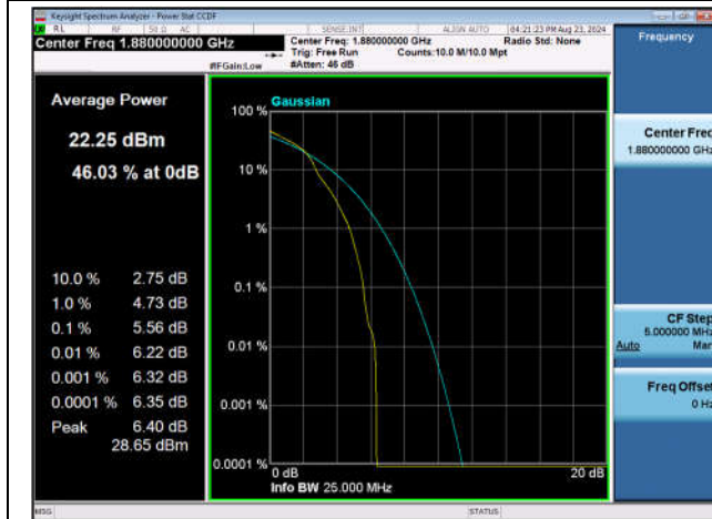
Band2-20MHz-16QAM-18900-1RB#0-PASS
