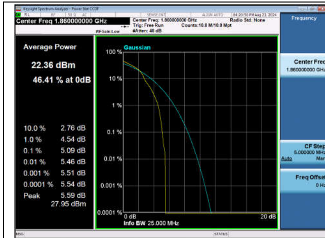
Band2-20MHz-16QAM-18700-1RB#0-PASS
