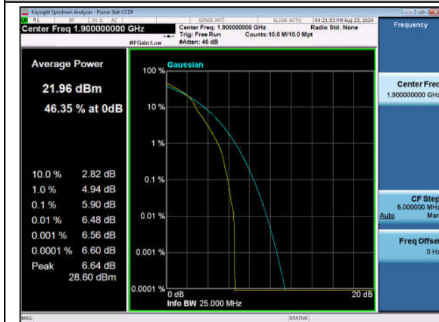
Band2-20MHz-16QAM-19100-1RB#0-PASS
