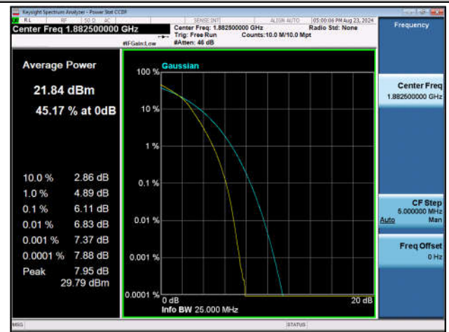
Band25-20MHz-16QAM-26365-100RB#0-PASS
